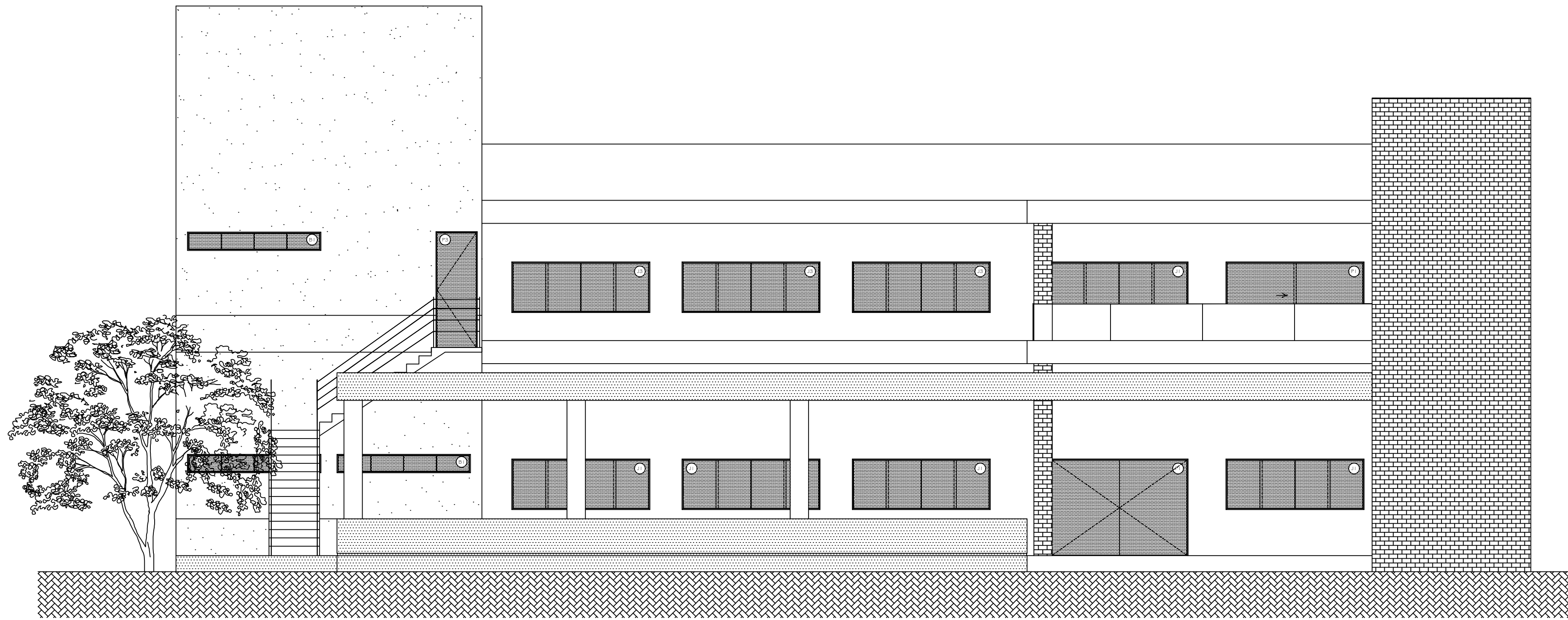
9 FACHADA ESCALA 1/50
