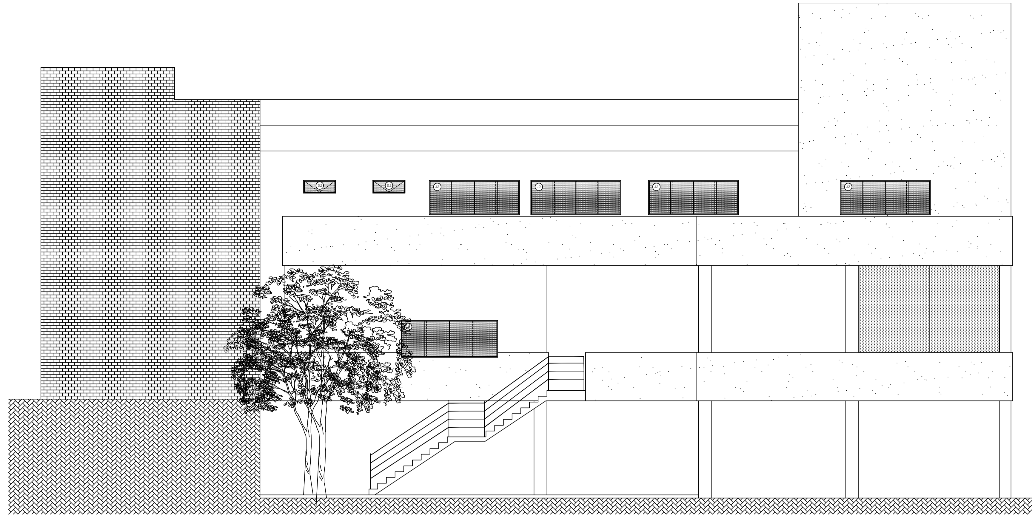
11 FACHADA ESCALA 1:50
