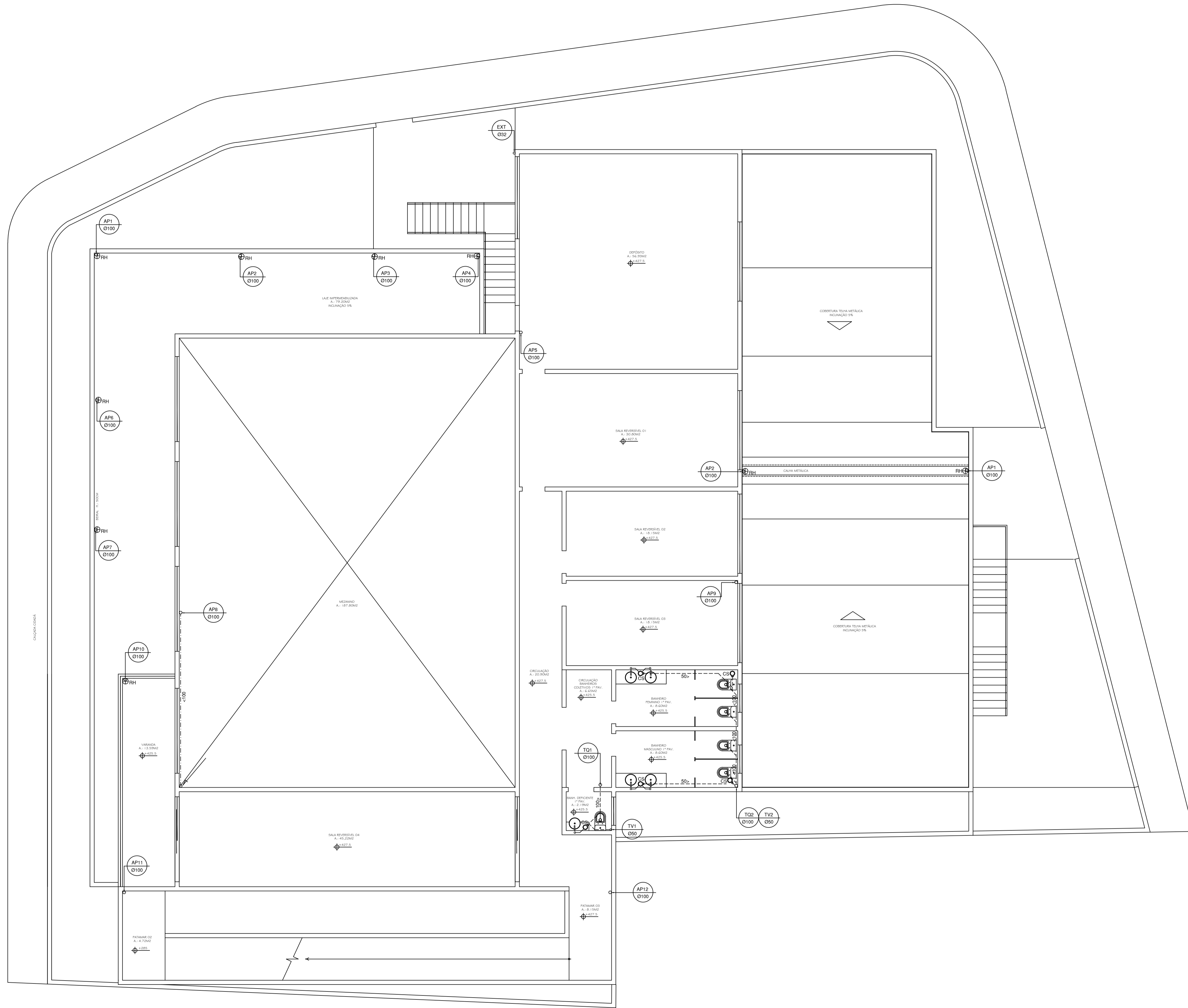
1º PAVIMENTO - REDE DE ESGOTO E DRENAGEM PLUVIAL PLANTA: BANHA ESCALA: 1/50
