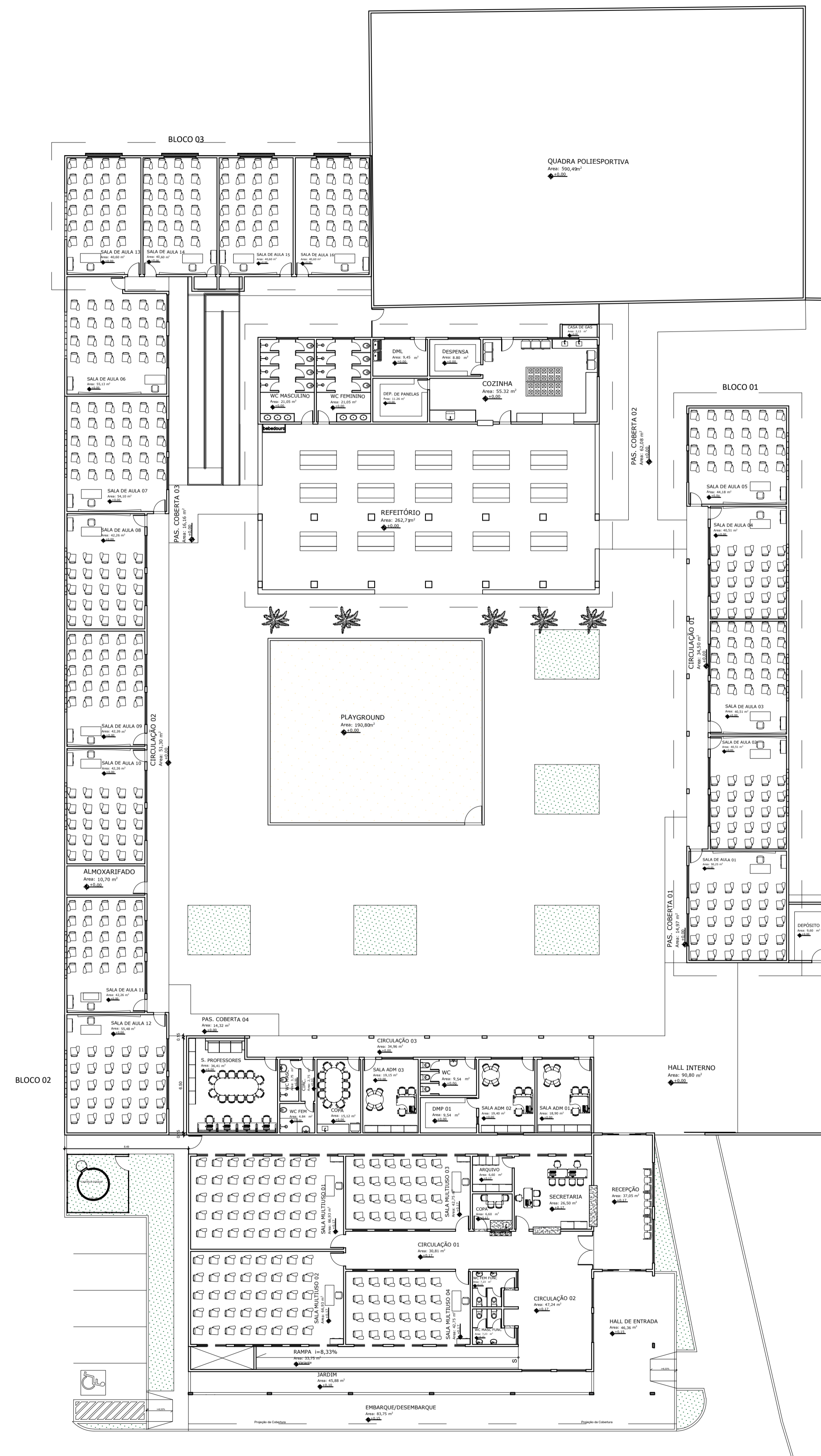
PLANTA DE LAYOUT- TÉRREO Esc. 1:200
