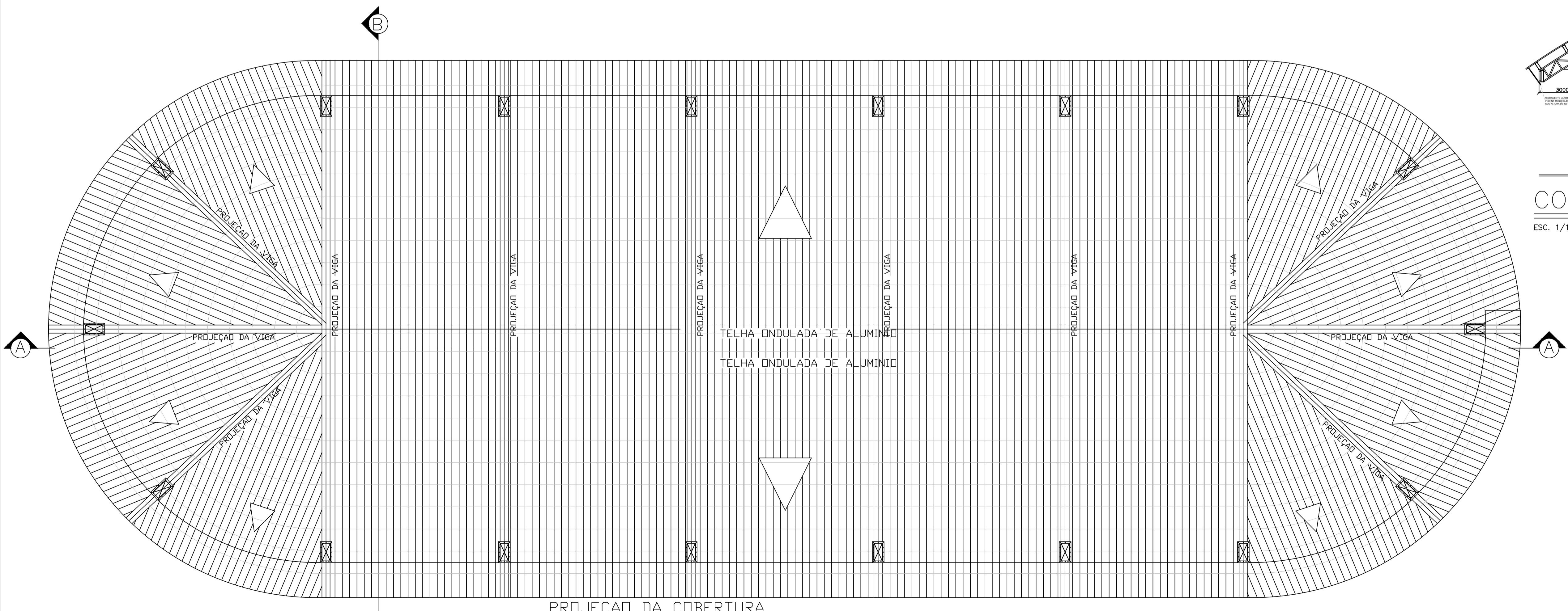
PLANTA DE COBERTURA
