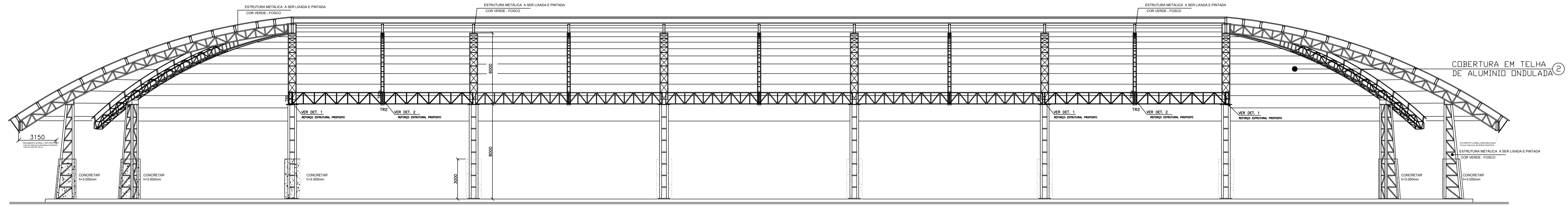
CORTE AA ESC. 1/150
