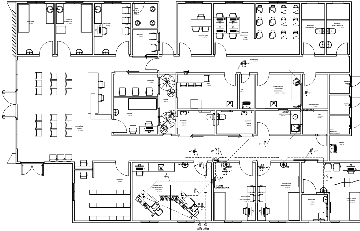
PLANTA BAIXA - TERREO (CAIXAS ODONTOLÓGICAS, TORNEIRAS ELÉTRICAS E AUTOCLAVES) ESCALA 1:60
